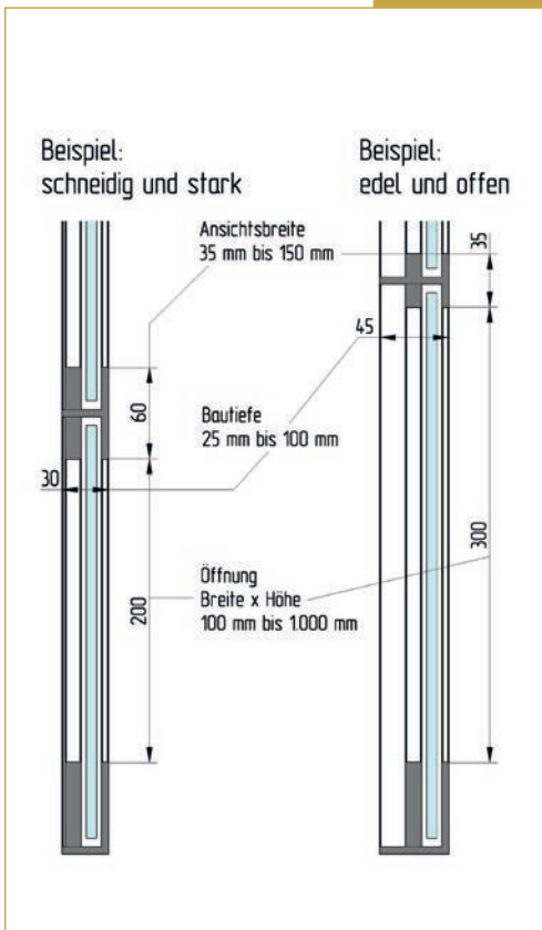
Beispiele Sprossenteilung & Systemschnitt
