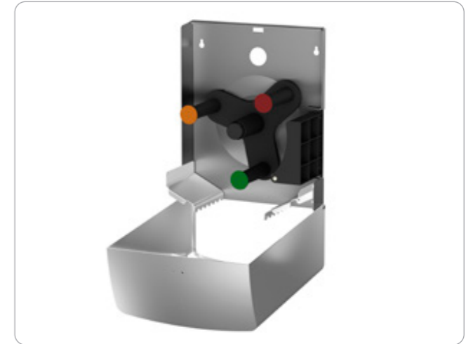
Spender mit Haushaltsrollen-Adapter und Rollenstopper.
